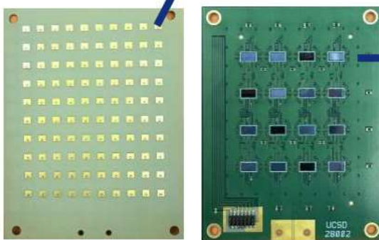
64 Antenna Array
